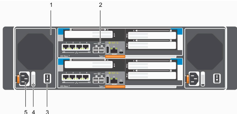
图 2: SC7020 存储系统背面板视图
